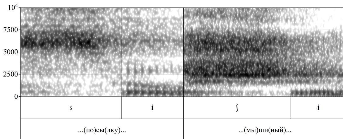
Рис. 1. Спектрограммы [с] и [ш], иллюстрирующие типичное соотношение (первых) частотных пиков в речи одного и того же респондента (АА-06)
